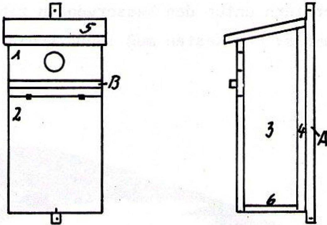
Abbildung 28: Bauanleitung Bilchkasten, Quelle: NABU Rinteln
