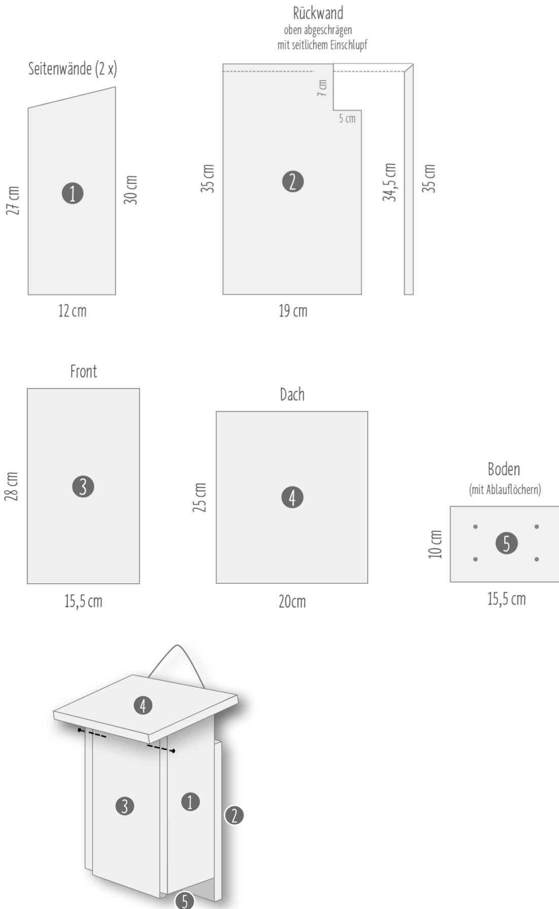
Abb. 16: Bauanleitung Baumläufer, Brettstärke 1,8cm. Quelle: NABU-Bundesverband, NABU (Naturschutzbund Deutschland) e.V.
