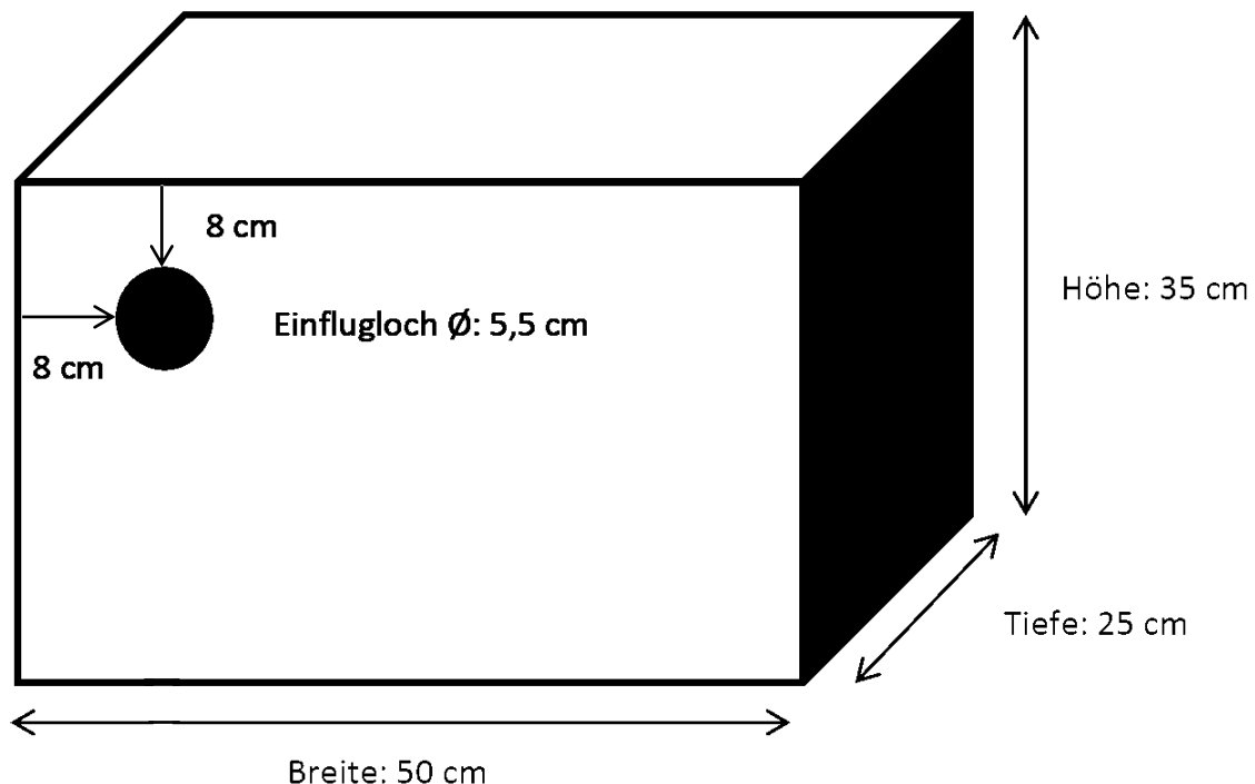
Abb. 6: Anleitung Maßangaben Wiedehopfkasten. Quelle: Eckenfellner, M., https://www.hoopoe.world/
