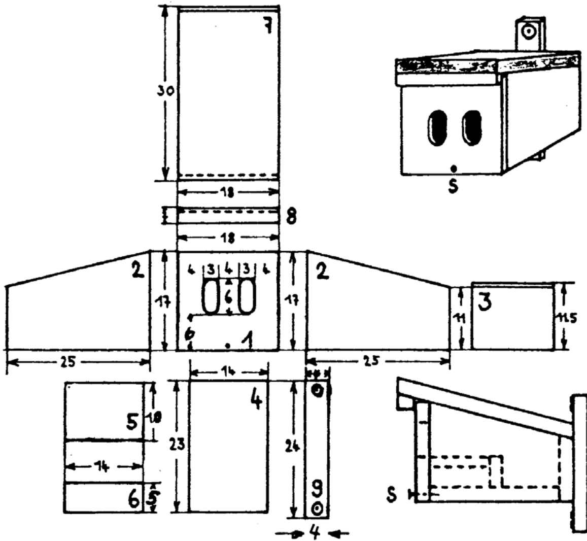
Abb. 10: Bauplan für eine Geschlossene Halbhöhle, Angaben in cm. Quelle: Morawski, E. (2004): Bauplansammlung von Nistkästen und Wohnhöhlen für Vögel, Insekten und Kleinsäuger. Eigenverlag NABU.
