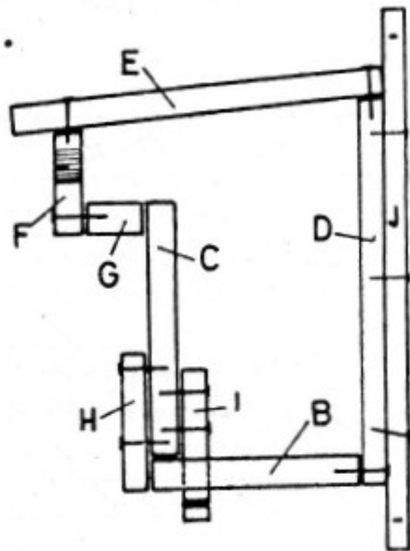
Abb. 14: Bauplan für Wendehalskasten, Quelle: NABU Rinteln
