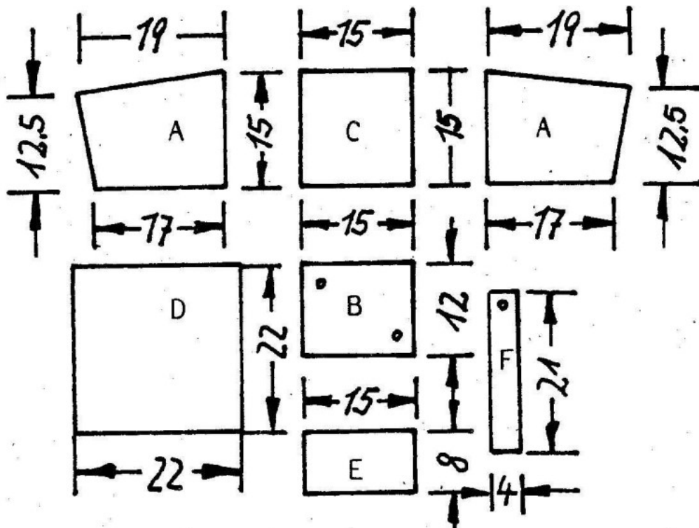
Abb. 12: Bauplan für eine offene Halbhöhle, Angaben in cm. Quelle: NABU Rinteln
