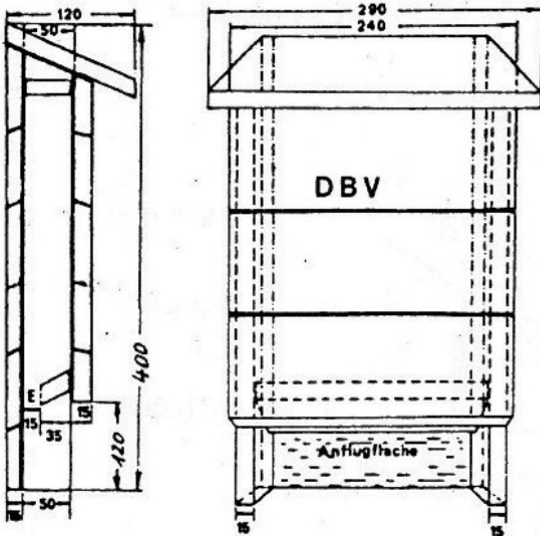
Abbildung 22: Bauplan für einen Fledermauskasten, alle Maßangaben in mm; Quelle: NABU Rinteln
