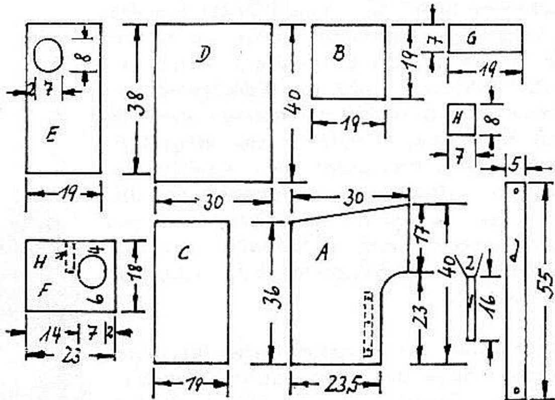
Abbildung 26: Bauplan für einen Raufußkauzkasten, Quelle: NABU Rinteln
