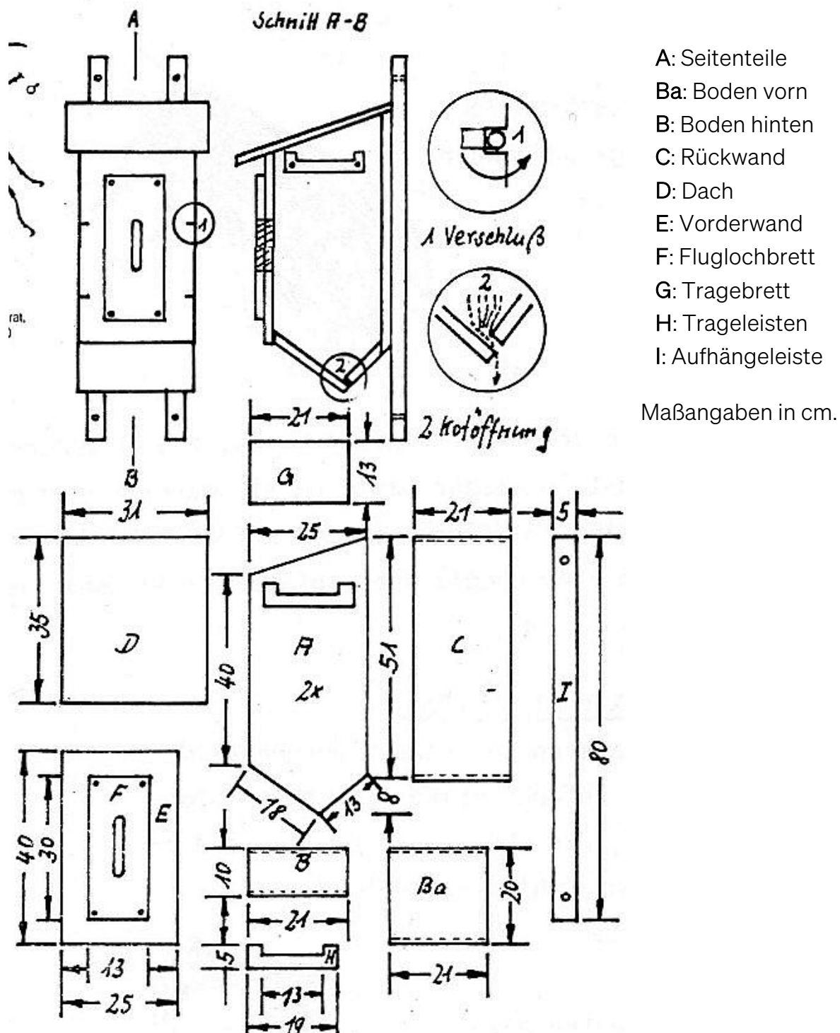
Abbildung 30: Bauplan für einen Hornissenkasten, Quelle: NABU Rinteln.
